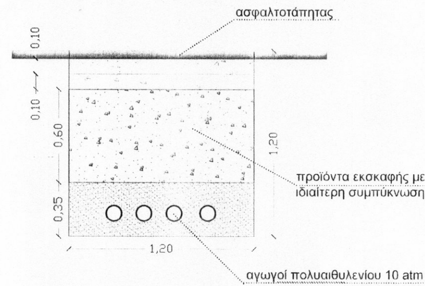
τομή εκτός οικισμού (ασφαλτόστρωση)
