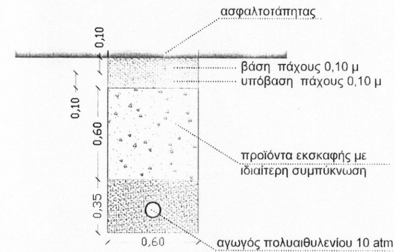
τομή εκτός οικισμού (ασφαλτόστρωση)
