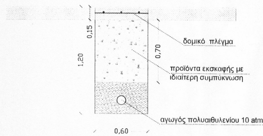
τομή εντός οικισμού (τσιμεντόστρωση)
